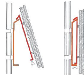
Einhängeprinzip der “MaEasy”
